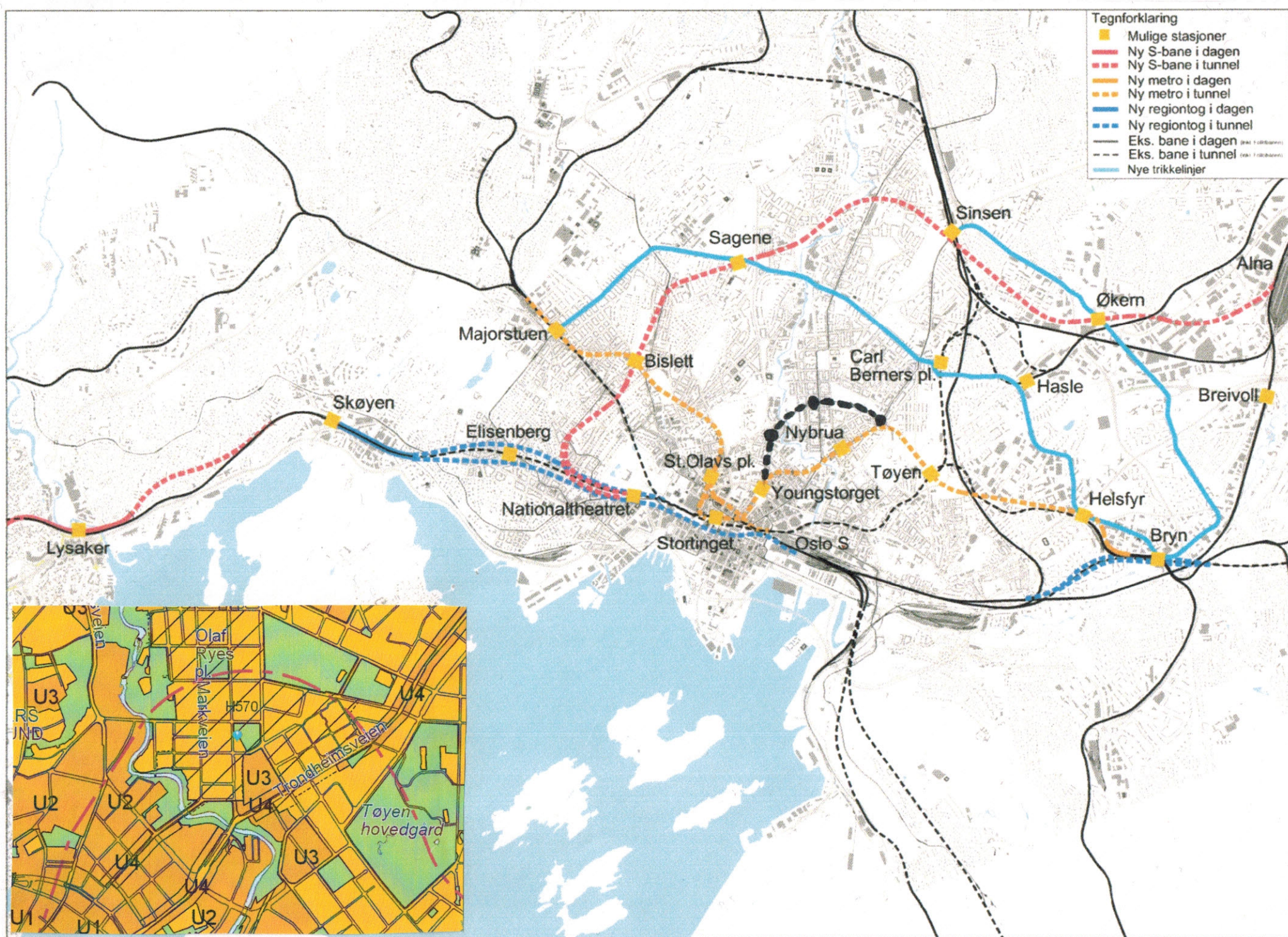
Figur 23: Oversiktstegning for anbefalt konsept K3A.
